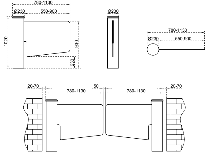
Ölçüler (mm)
