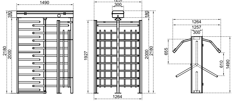
Ölçüler (mm)
